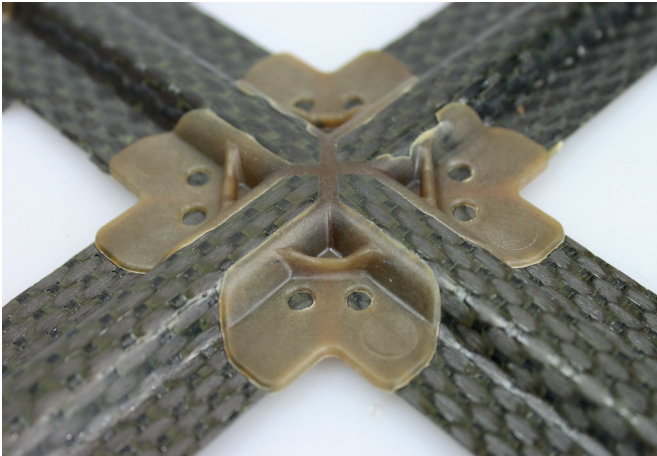
Detailaufnahme einer hybriden Versteifungsstruktur auf Basis von Polyetherimid (PEI/CF-GF)
