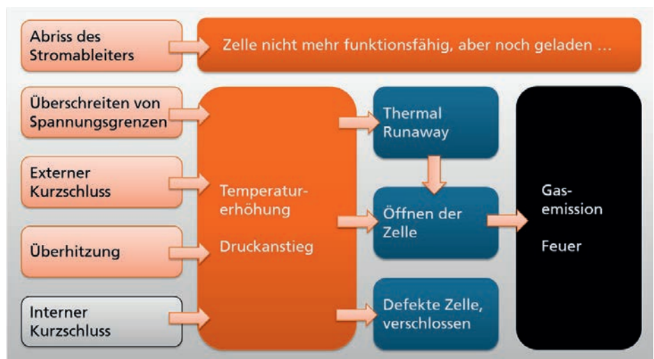
Mögliche Ausfallursachen an Lithium-Ionen-Zellen.
